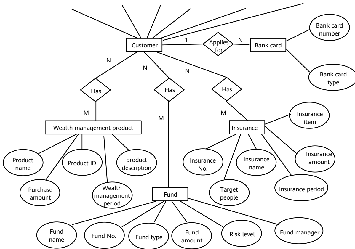
Figure 5-1 ER diagram
